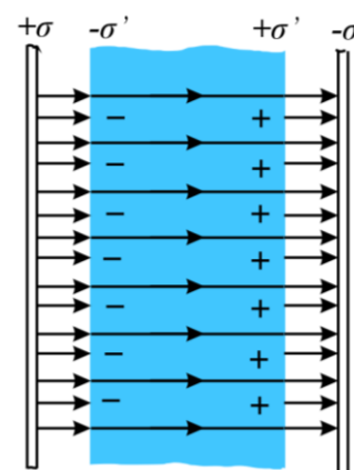
Рис. 4. Поле в диэлектрике
