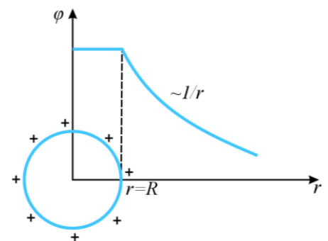
Рис. 3. Потенциал сферической поверхности
